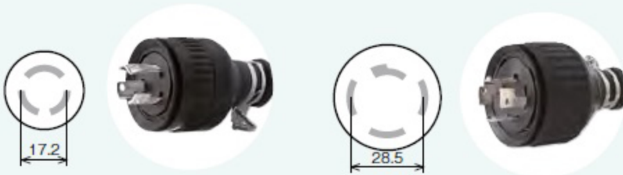
3極引掛形 15A 125V
