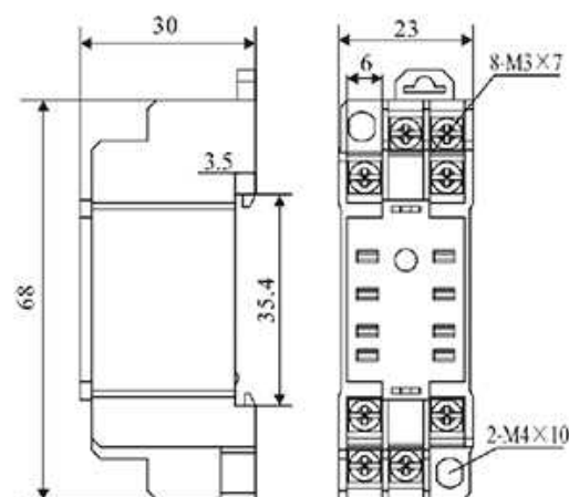
外形图 Outline
