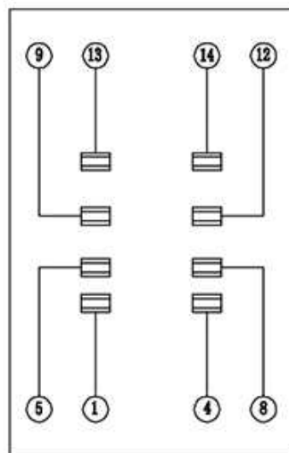
接线口 Wiring diagram
