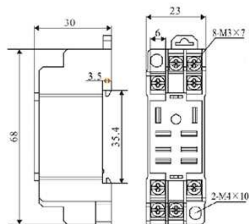
外形图 Outline
