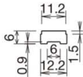
脱扣杆的文字记名板尺寸
