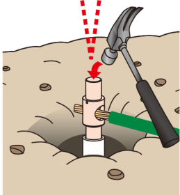
2 リード端子の打込みと同時に 接地線との接続が可能
