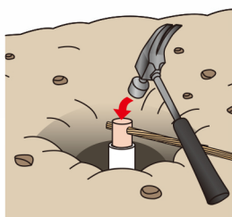
2 リード端子打込み
