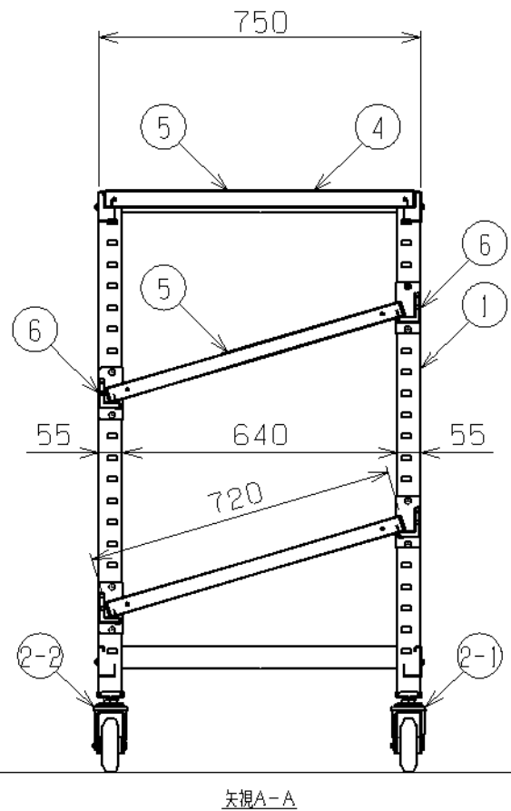
矢視A-A
