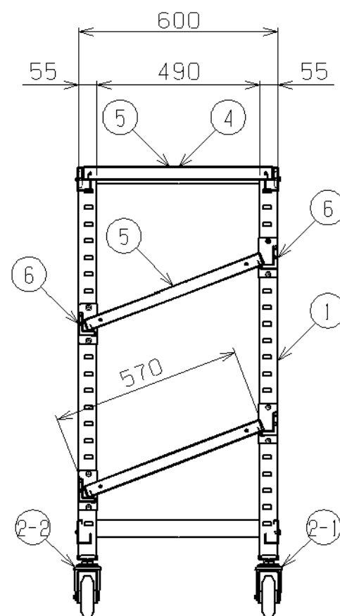
矢視A-A
