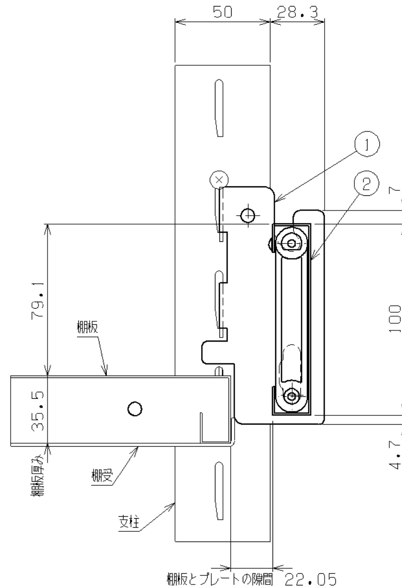
矢視A-A (セット時)
