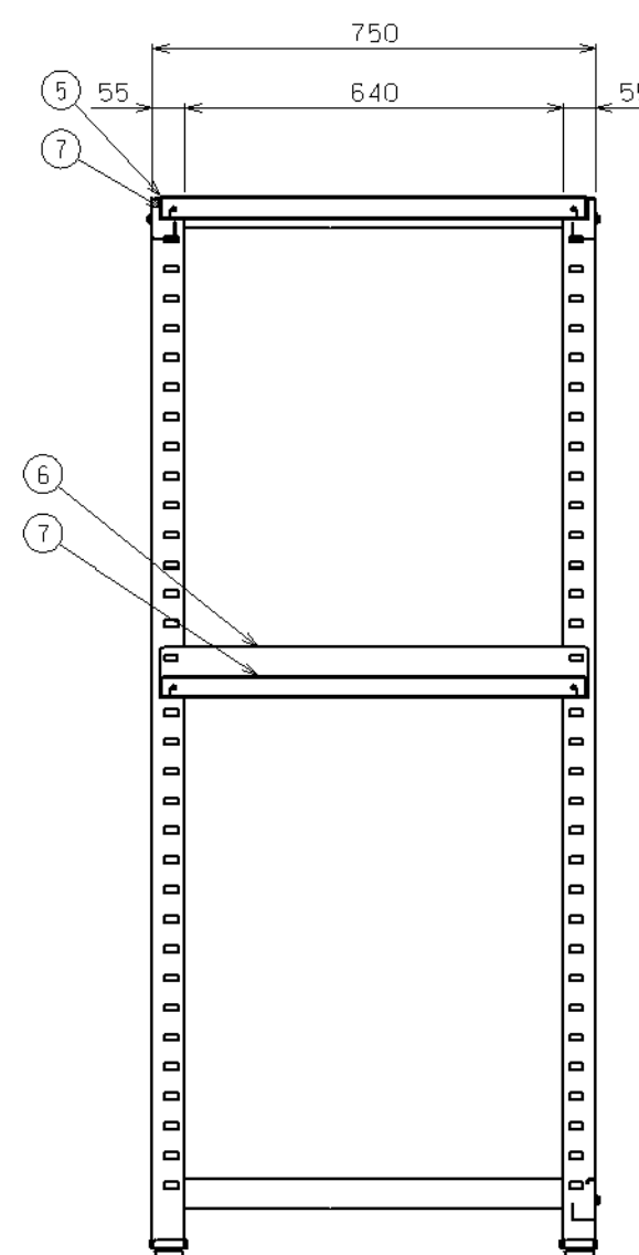
矢視A-A
