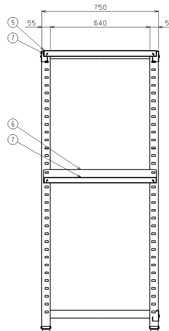
矢視A-A
