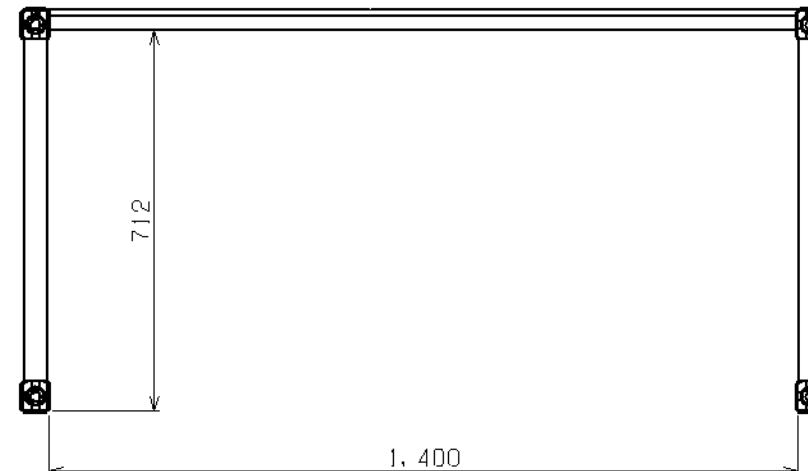
矢視B-B (下開放部詳細)
