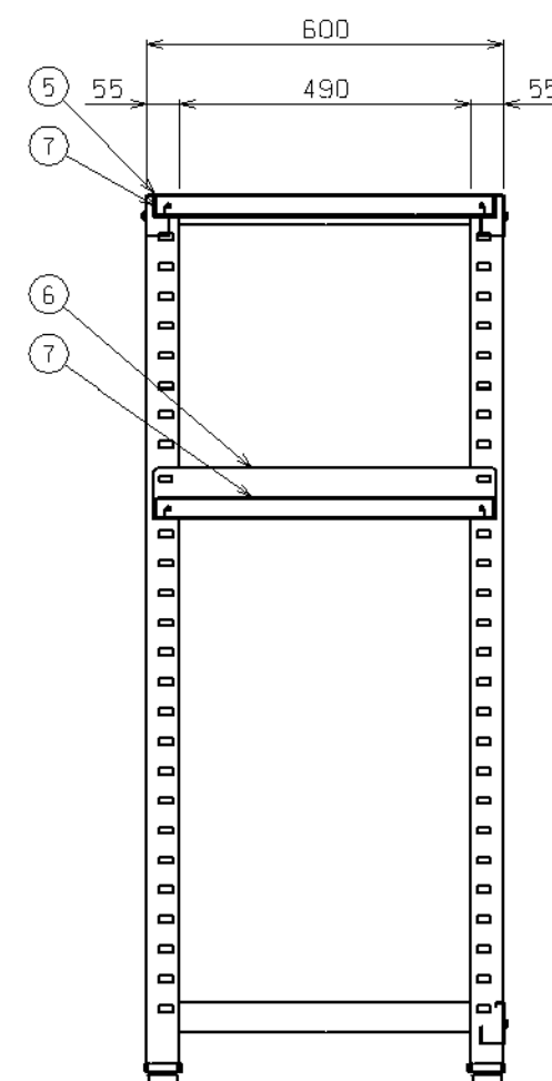
矢視A-A
