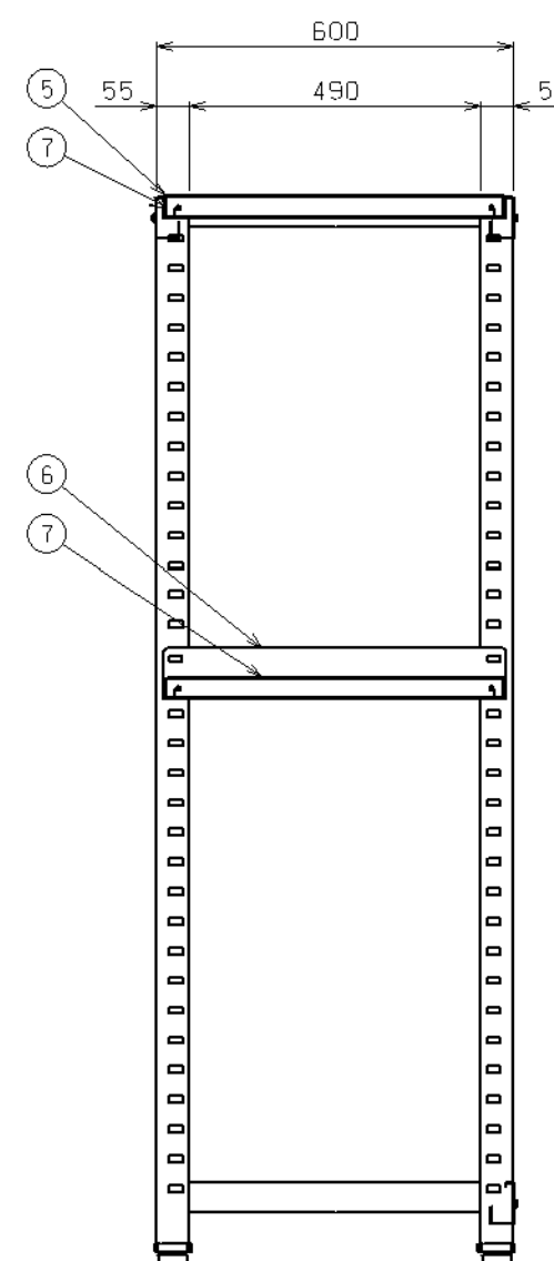
矢視A-A
