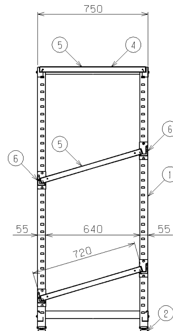
矢視A-A
