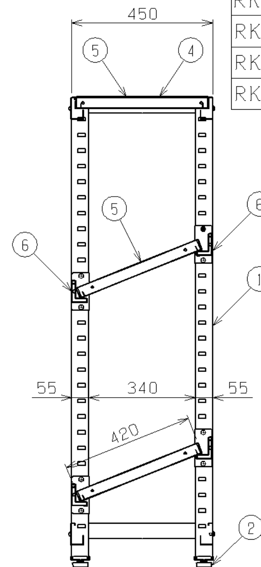
矢視A-A
