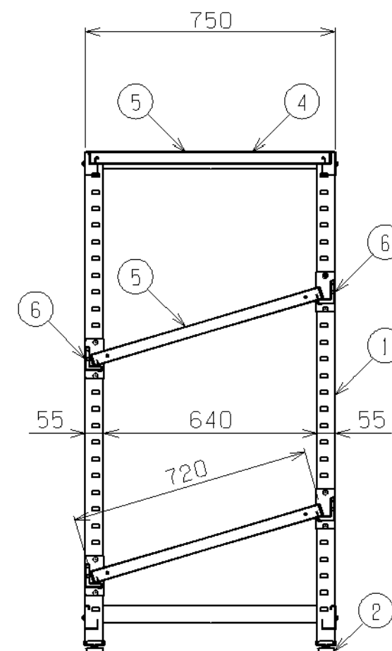
矢視A-A
