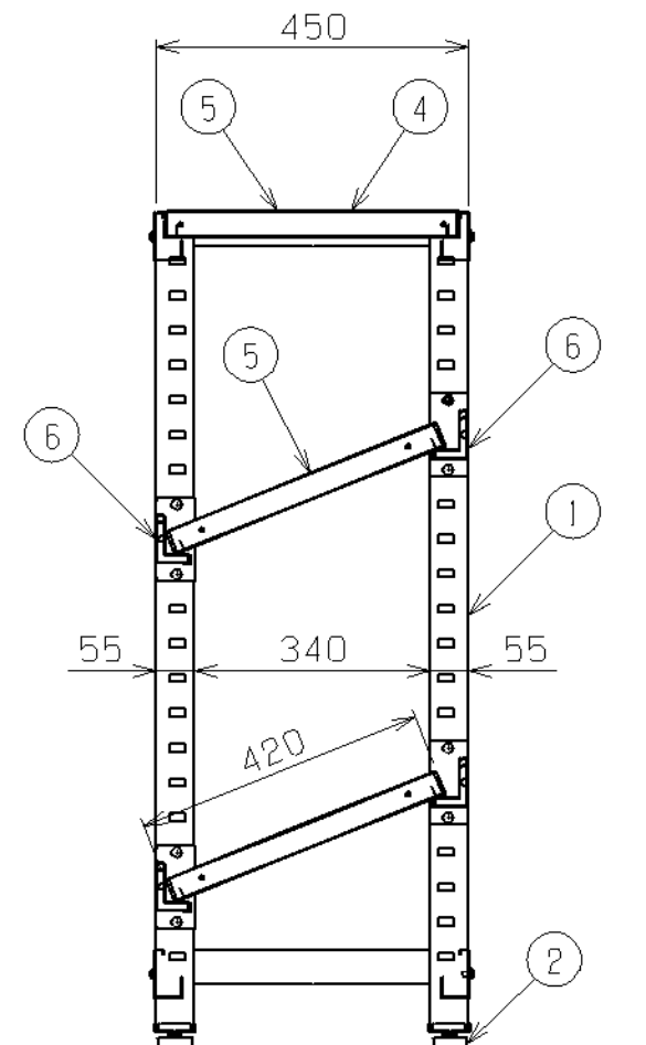
矢視A-A
