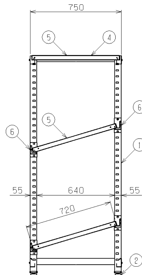
矢視A-A
