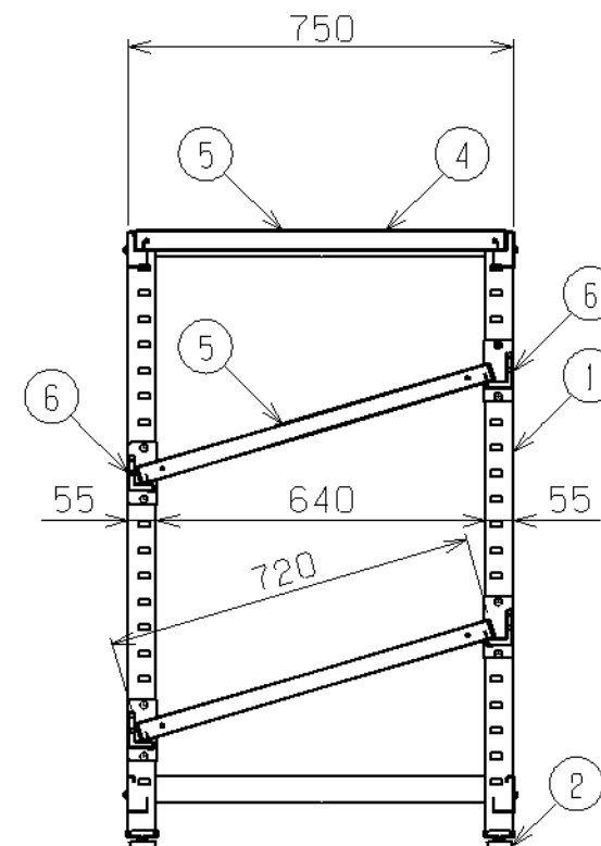
矢視A-A
