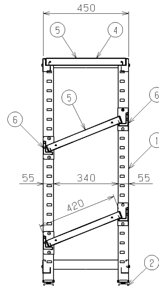
矢視A-A
