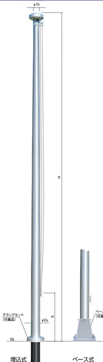
埋込式
