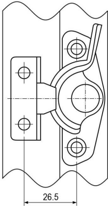
取付例 Installation Example
