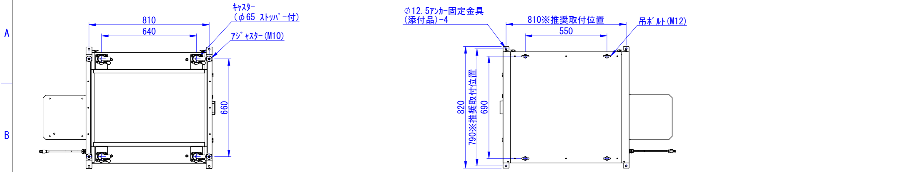
底面
