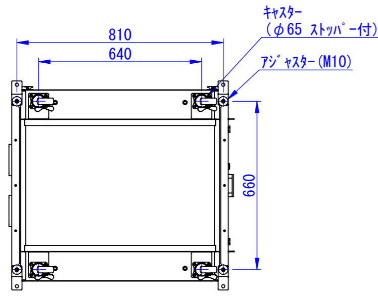
底面
