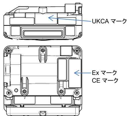
ATEX,IECEX,UKEX 仕様の銘板例
