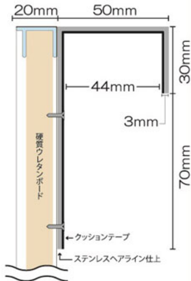
断面図
