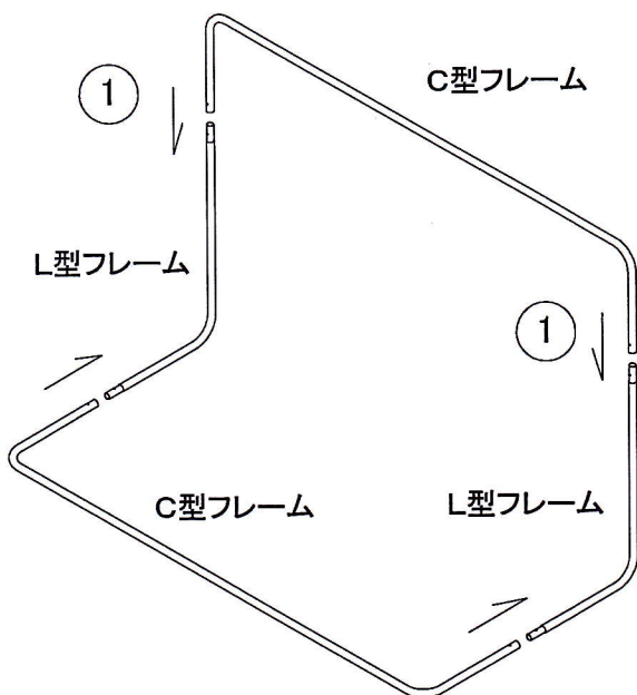
組立図
