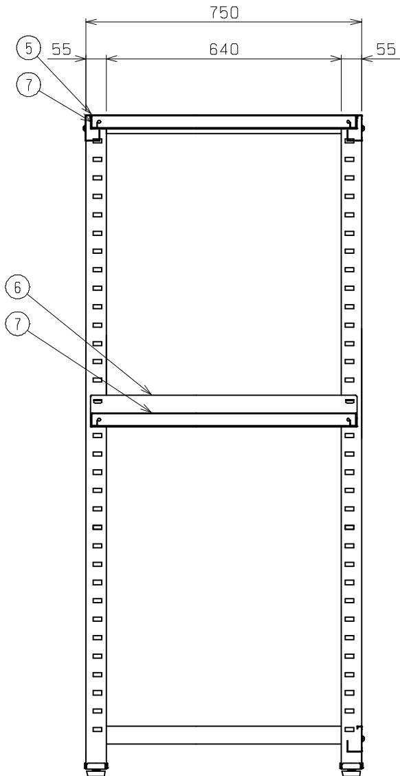
矢視A-A
