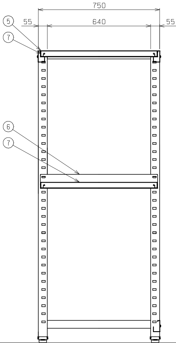
矢視A-A
