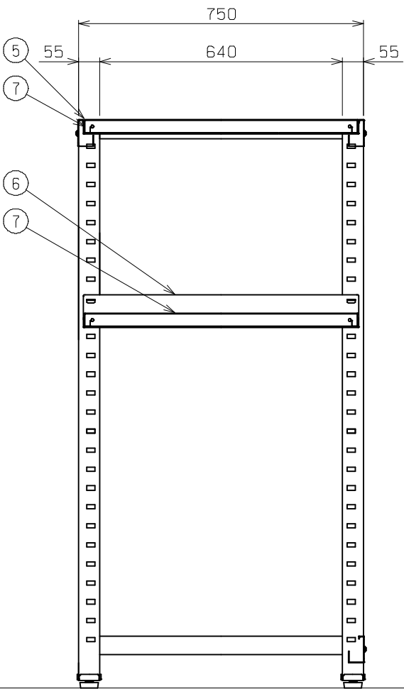
矢視A-A
