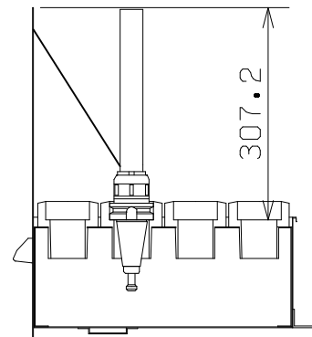
ツーリング引出し断面 AS-40用(品番Cタイプ)
