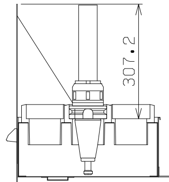
ツーリング引出し断面 AS-50用(品番Aタイプ)
