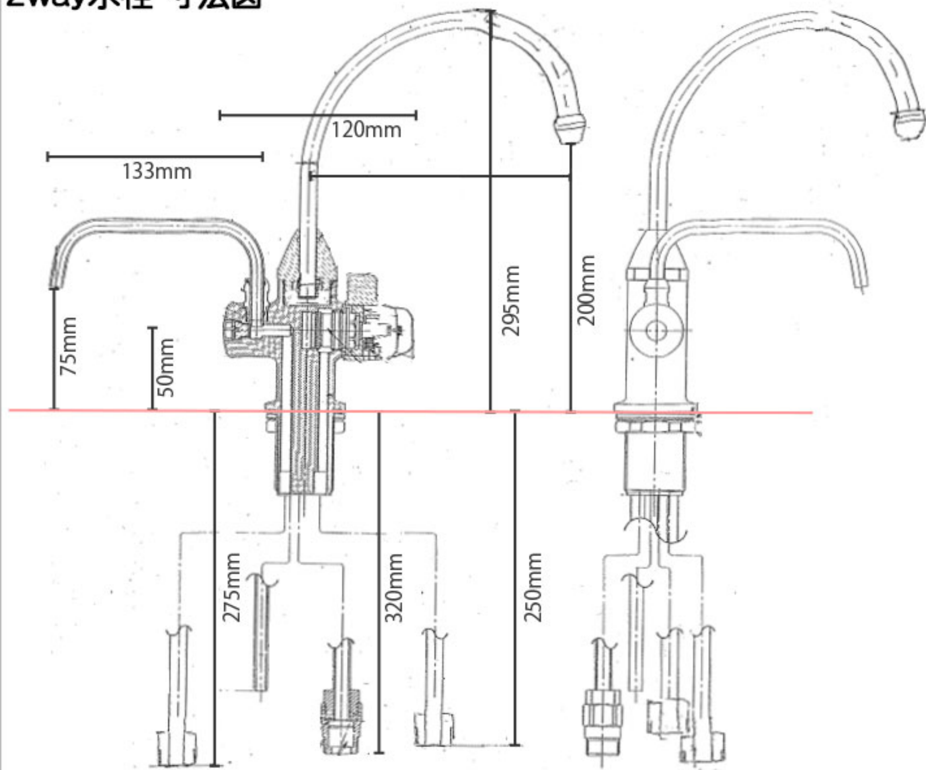
2way水栓 寸法図
