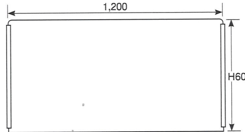
1,200×H600 (切込み無) E110-205-50 (3mm厚) (板のみ)
