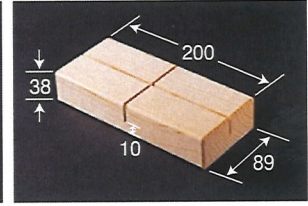
パーティション用木製受台 E110-206-50 (大) 1個
