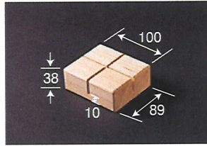
パーティション用木製受台 E110-206-40 (小) 1個
