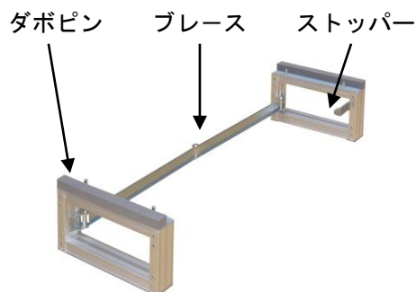
③ 開いた枠に段板をセットします。
