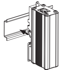
DINレール取付例 (DIN規格 35mm幅)
