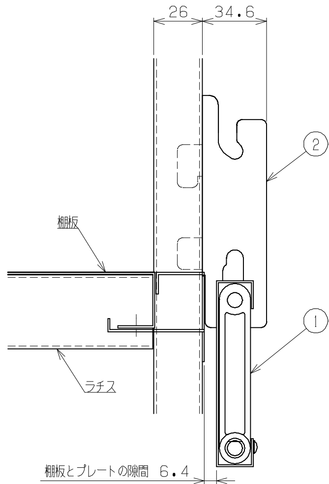
矢視A-A（解除時）
