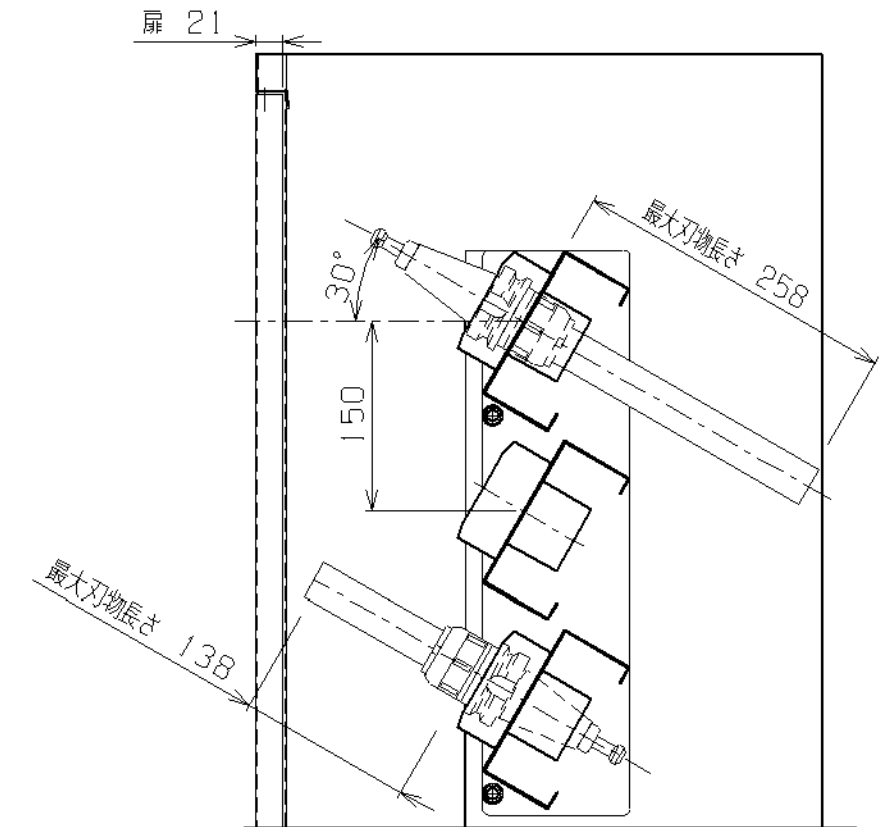
ツーリングホルダー詳細 (S=1/6)
