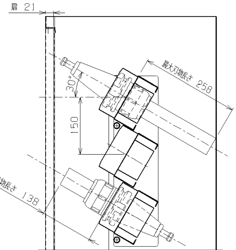
ツーリングホルダー 詳細 (S=1/6)
