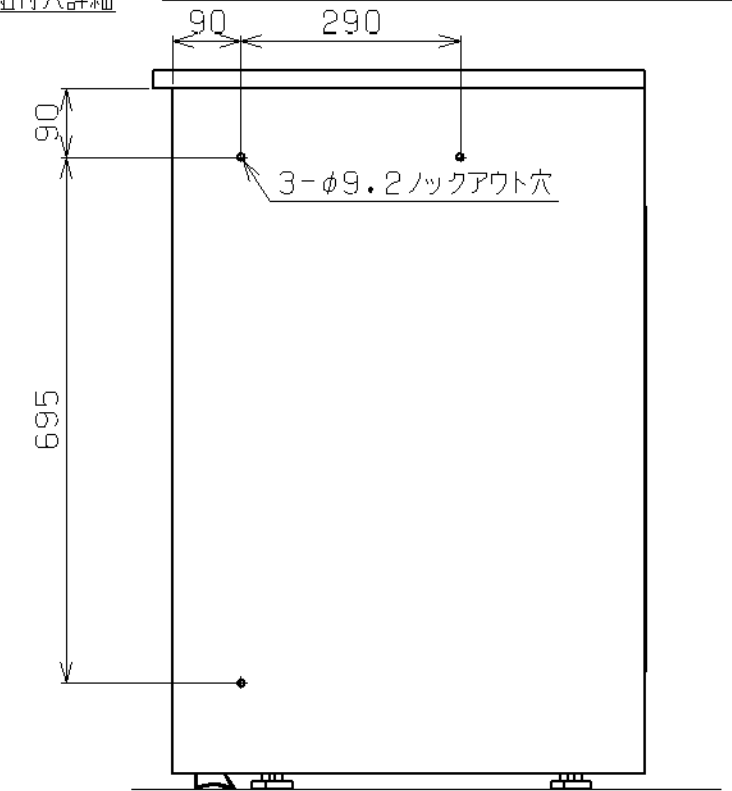
組付穴詳細
