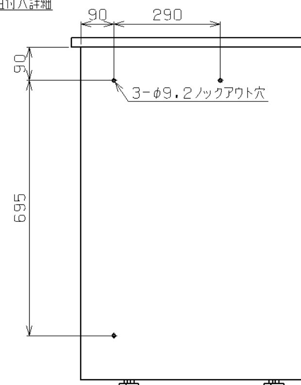
組付穴詳細
