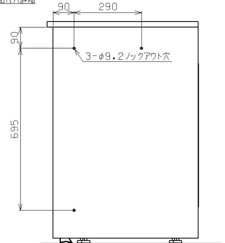
組付穴詳細
