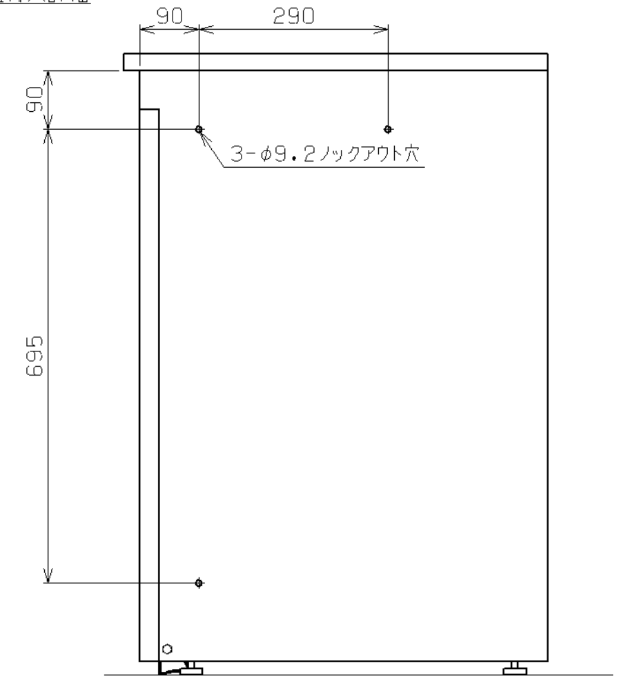
組付穴詳細
