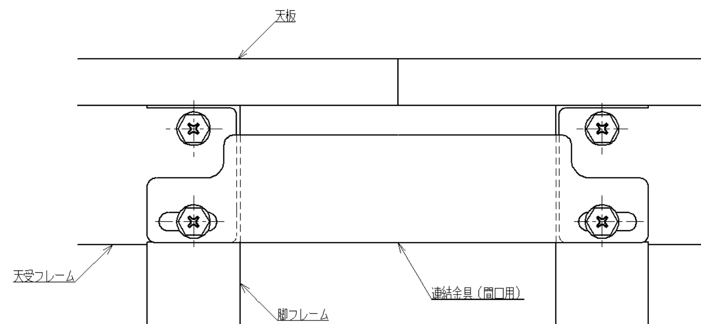
取付詳細図
