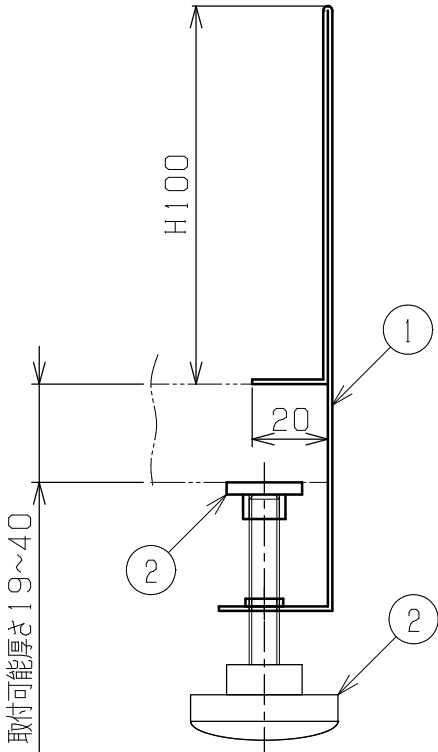
天板取付詳細 (S=1:2)
