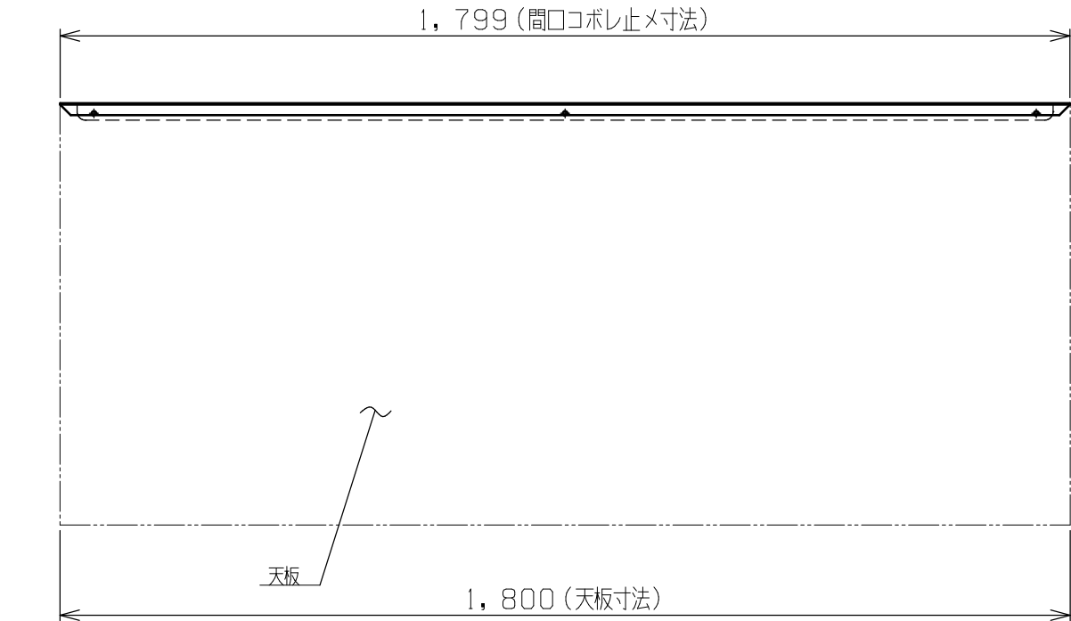
取付例 (S=1:12)
