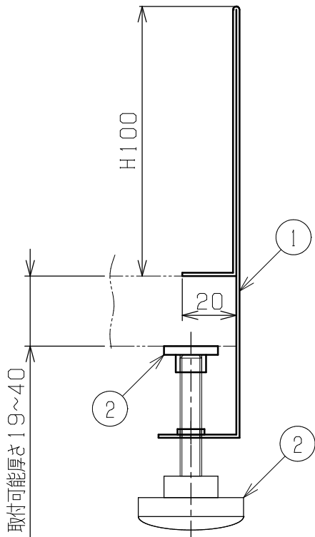
天板取付詳細 (S=1:2)
