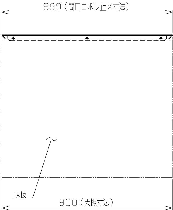
取付例 (S=1:12)
