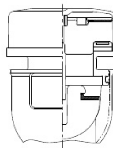
組立図（開時）
