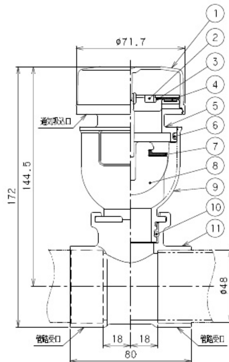
組立図（閉時）
