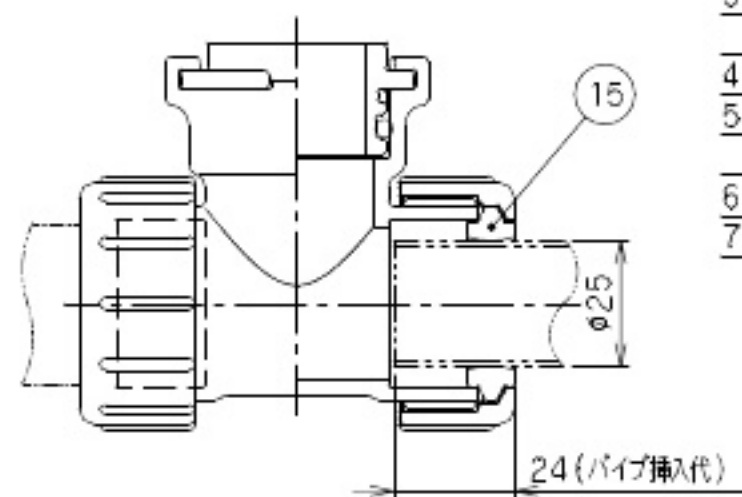
呼び径25
