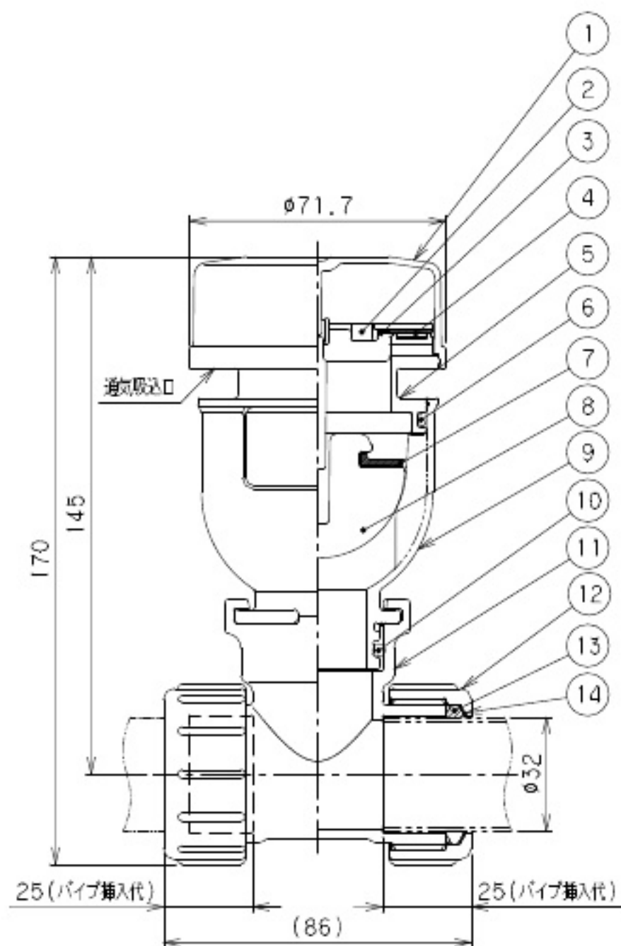
組立図(閉時)
