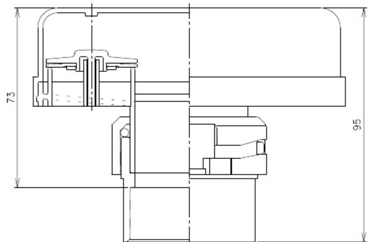
組立図
