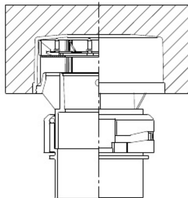
組立図 (開時)
