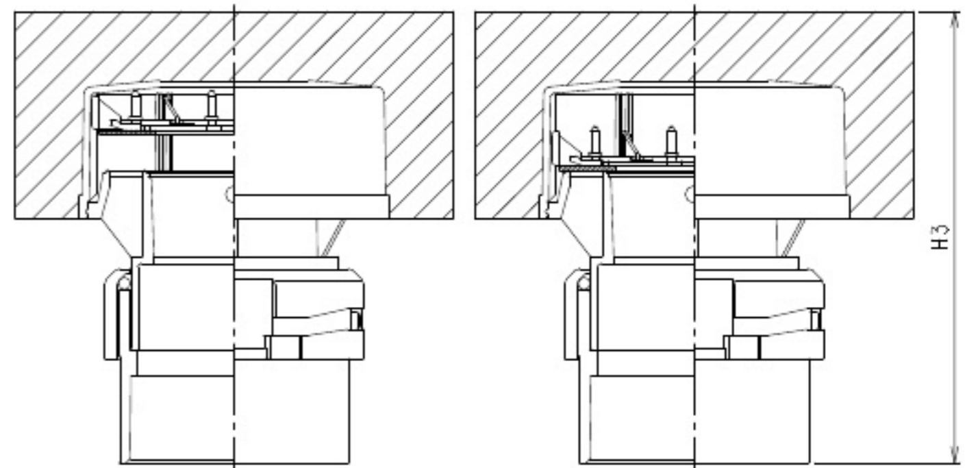
組立図 (開時)
